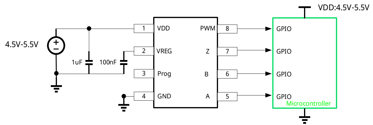
典型应用图
