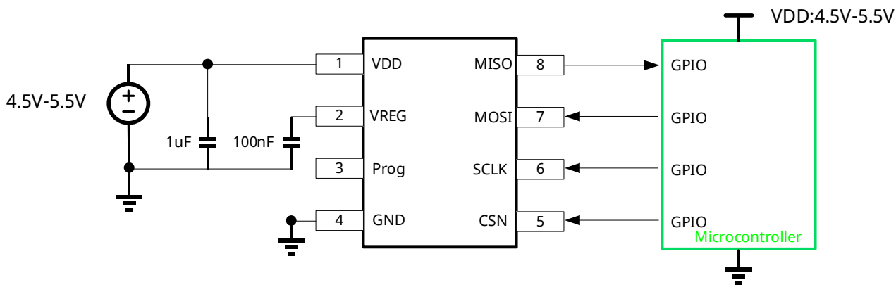
典型应用图
