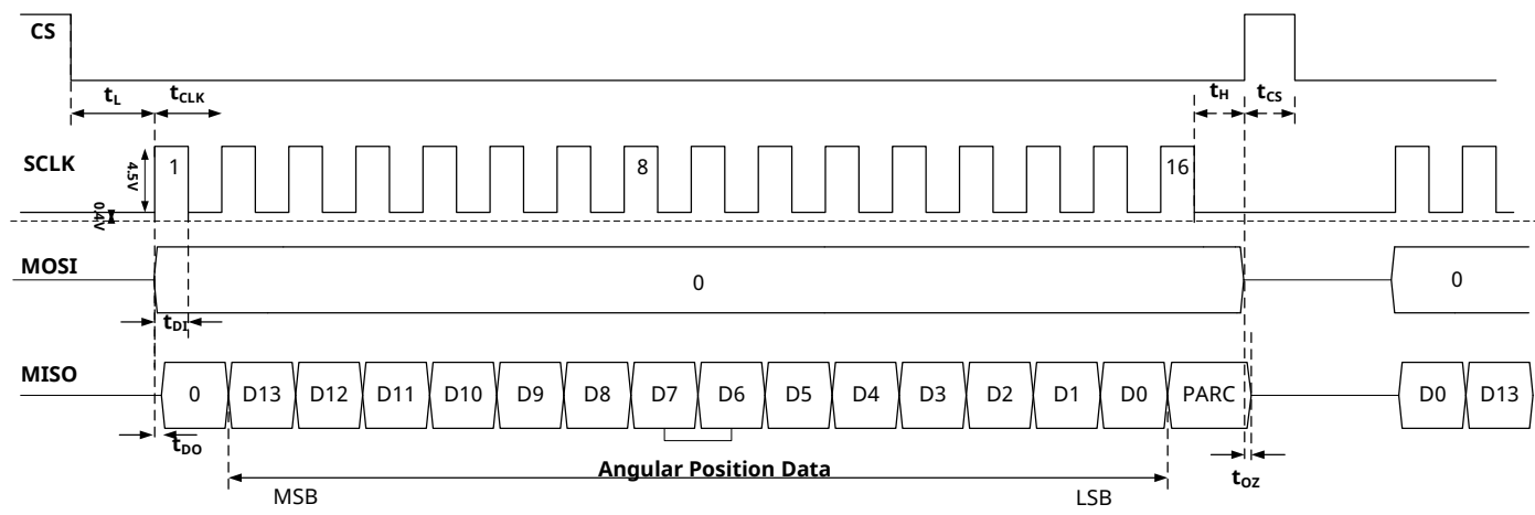
图 11 SPI 角度读取模式图
