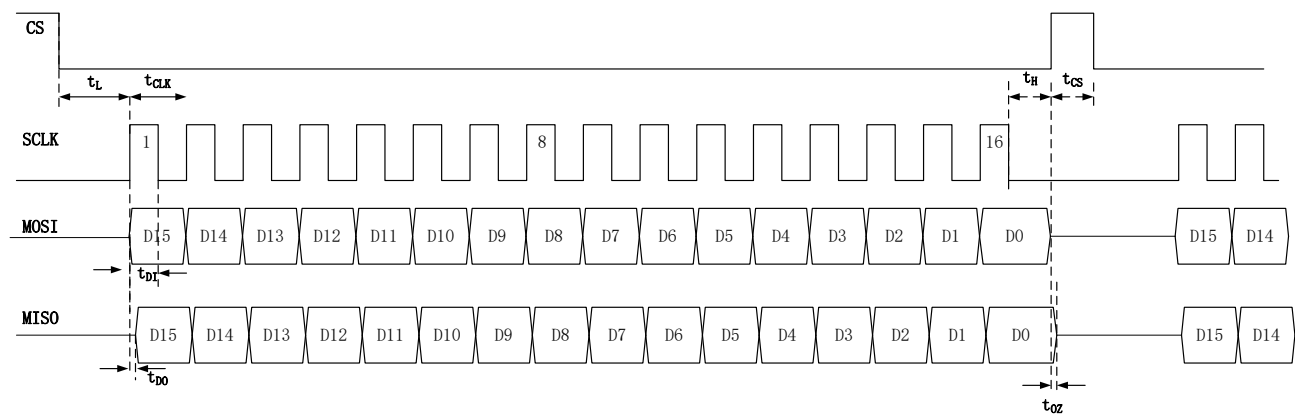
图 10 SPI 寄存器读写模式图
