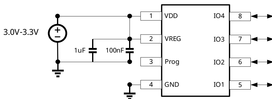
图 13 3.3V 供电电路图
