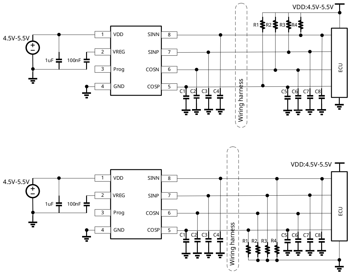
图 4 模拟输出应用图：上拉电阻配置(上)&下拉电阻配置(下)
