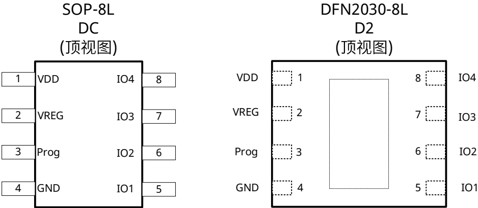
图 2 SOP-8L 封装顶视图(左)&DFN2030-8L 封装顶视图(右)
