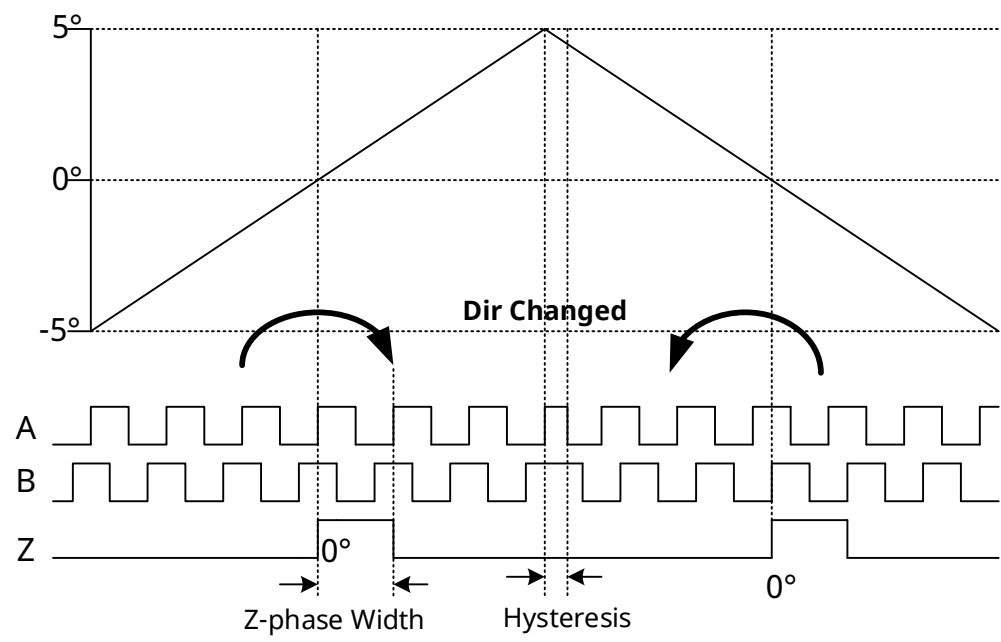
图 7 增量输出波形图
