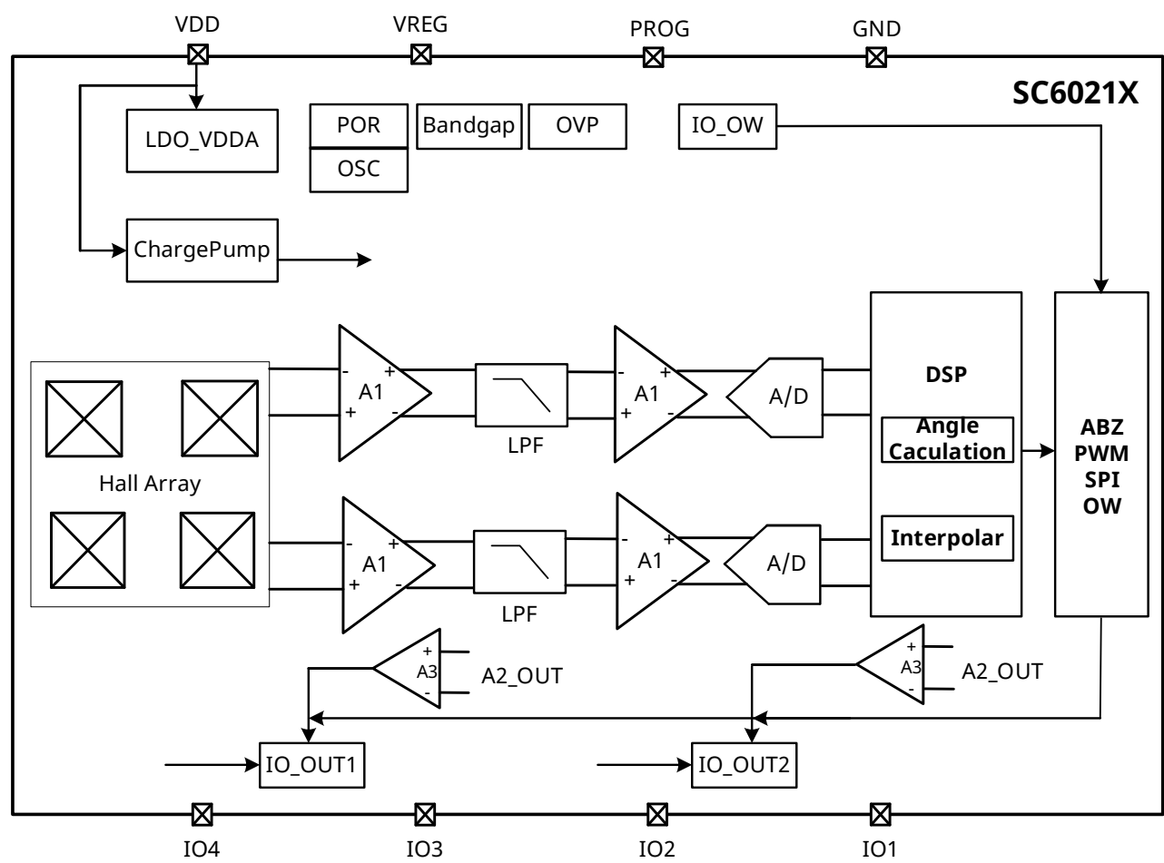
图 3 功能框图
